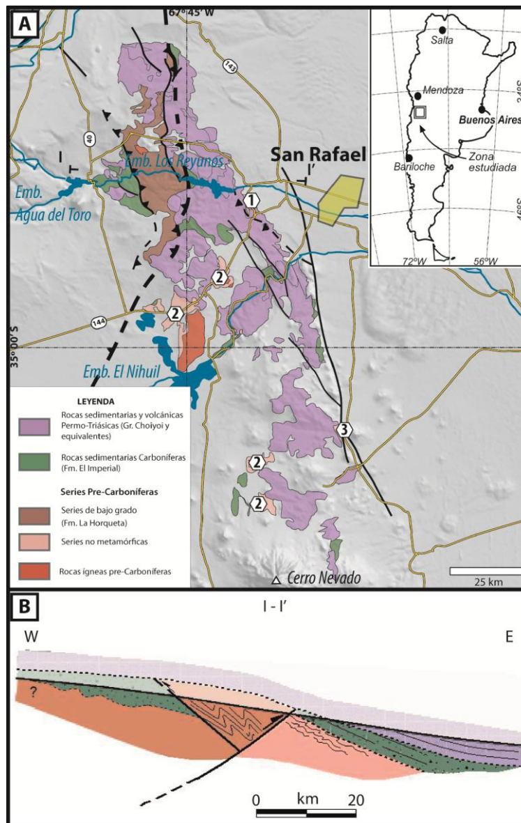
FIGURA 1. (A) Bosquejo geológico del Bloque San Rafael. (1) Fm. Pavón. (2) Fm. Río Seco de los Castaños. (3) Fm. Ponón Trehue, discordante sobre rocas del basamento Proterozoico. Basado en Sepúlveda et al. (2007a, b). (B) Corte geológico I-I' entre el Embalse Agua del Toro y 25 de Mayo.
